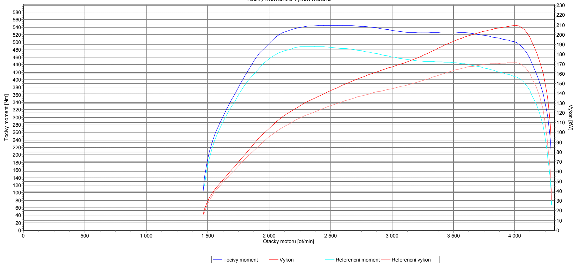
Tocivy moment a vykon motoru
