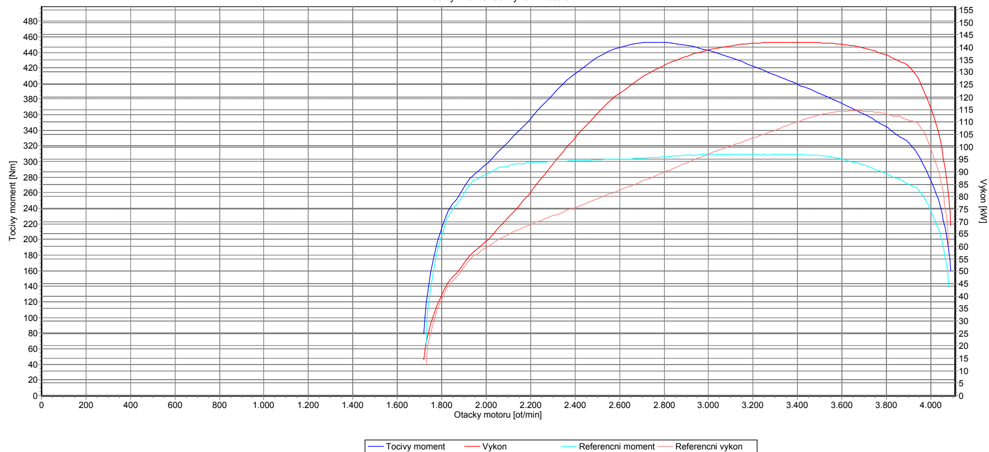
Tocivy moment a vykon motoru
