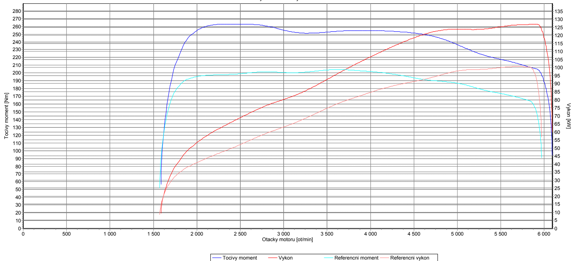
Tocivy moment a výkon motoru
