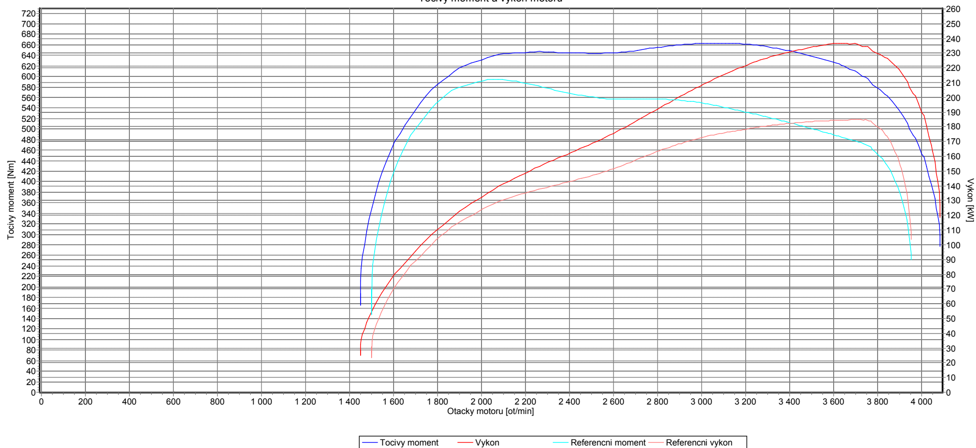
Tocivy moment a výkon motoru
